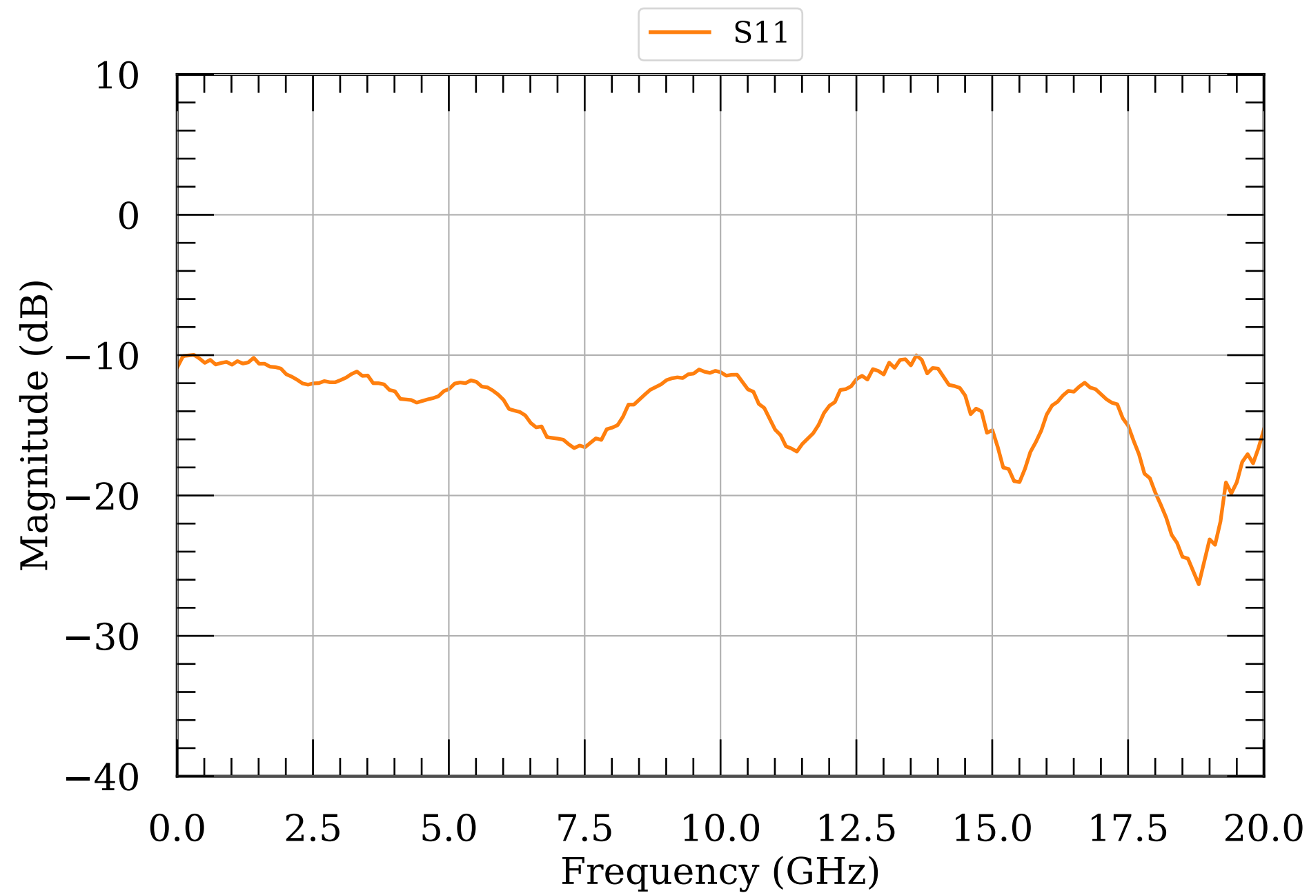
LNA S-params module032
